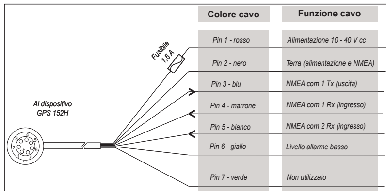
Conduttore di GPS 152H
